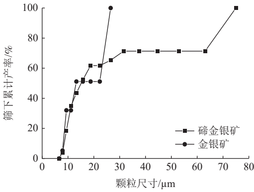
图 3 金矿物粒度分布曲线
