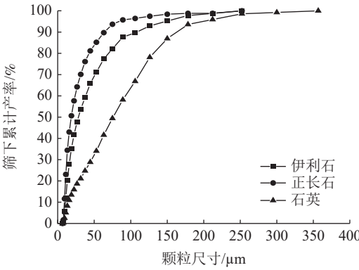
图 4 主要脉石矿物粒度分布曲线
