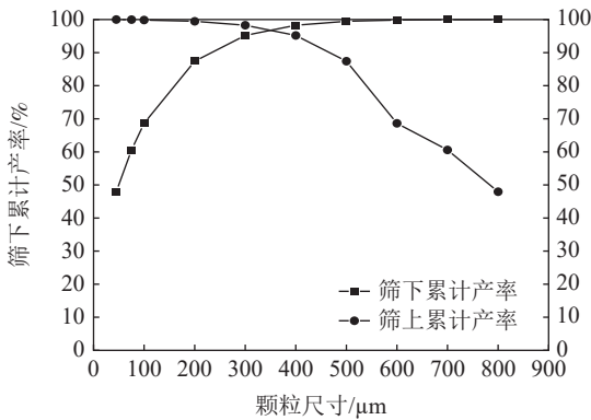
图 2 样品粒度分布曲线
